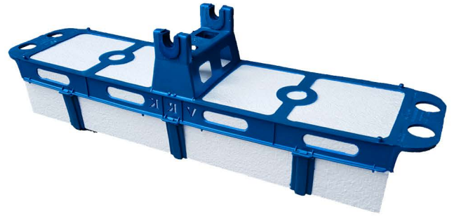
ทุ่น พร้อมโฟม 8 นิ้ว รหัส 123/1 325 x 1370 x 400 มม.
